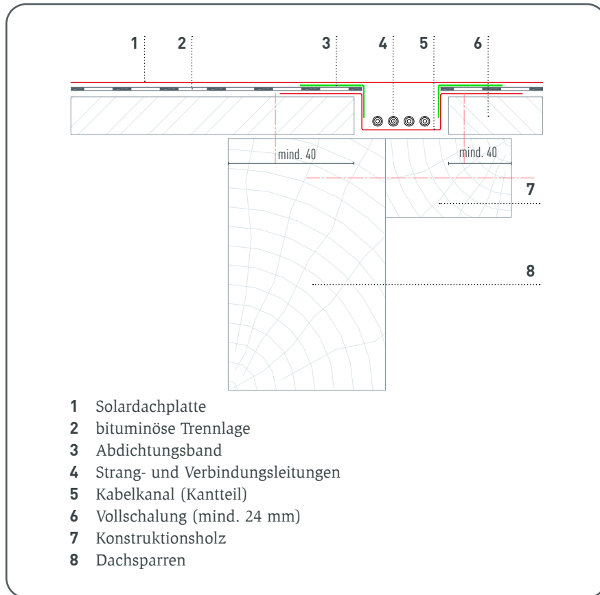
Abbildung 16 · Kabelkanal einschligig schmal
