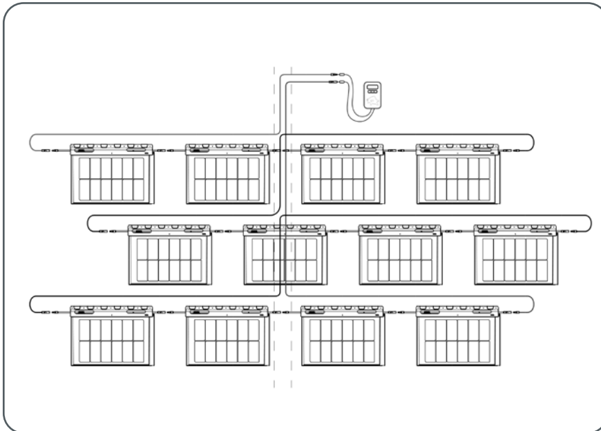
Abbildung 20 · Spannungsprüfung des Stranges
