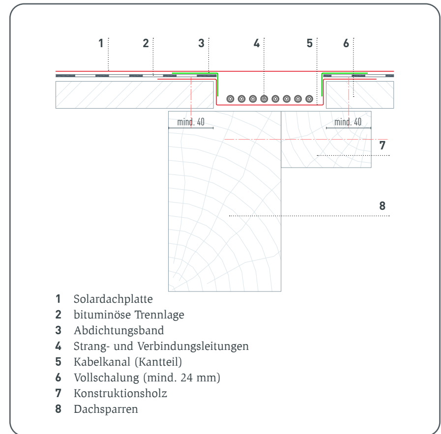
Abbildung 15 • Kabelkanal einschalig breit
