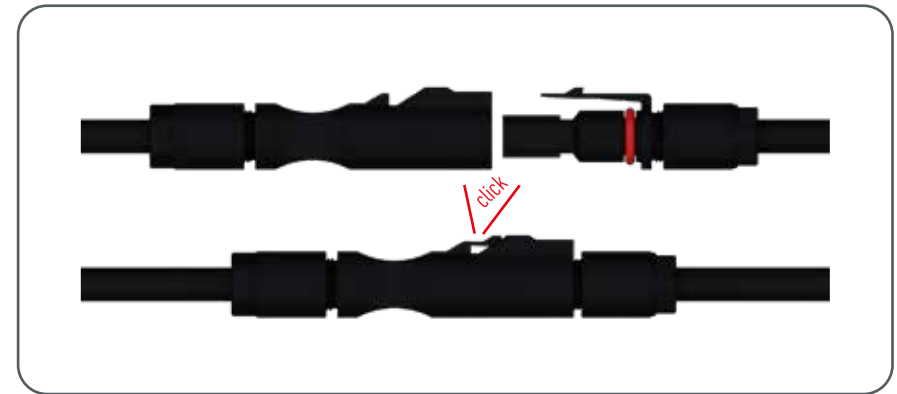
Abbildung 1 • Kontaktierung der Solarlok „Slim Line Stecker“
