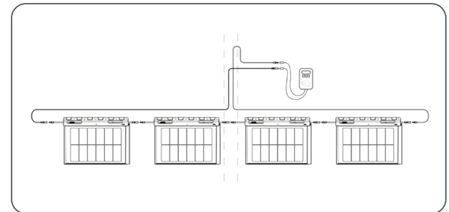
Abbildung 19 • Spannungsprüfung der Reihen
