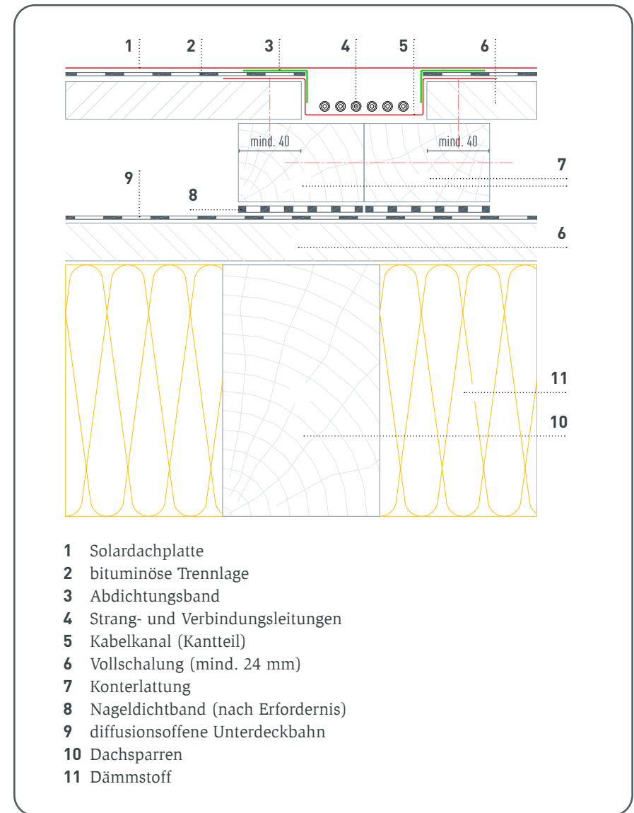
Abbildung 17 · Kabelkanal zweischligig breit
