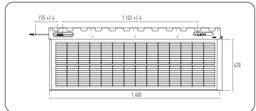
Abbildung 13 · Zeichnung Solardachplatte groß
