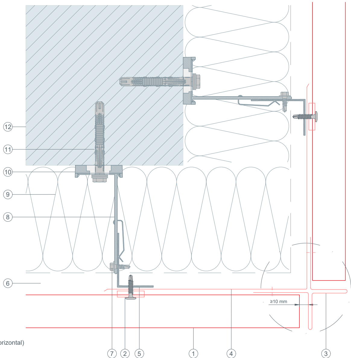
Anschlussvariante
