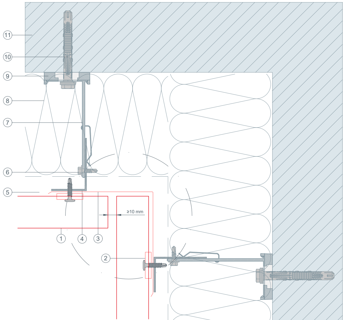
Anschlussvariante
