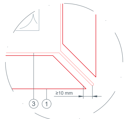
Anschlussvariante
