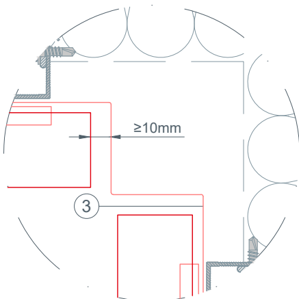
Anschlussvariante
