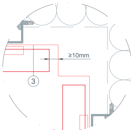
Anschlussvariante
