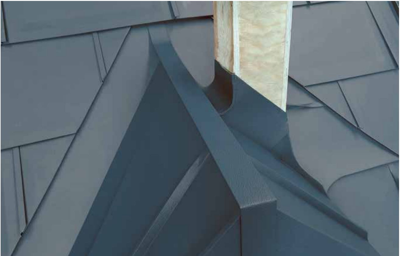
Einfassung eines Kamins in der Kehle
